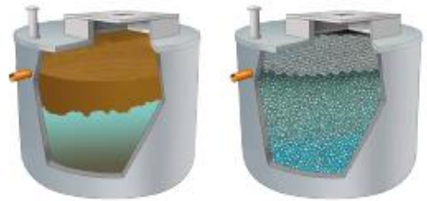
Gamme deux cuves BIOFRANCE® Passive
